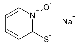
Pyridin-2-thiol-1-oxid, Natriumsalz (NaPt)
